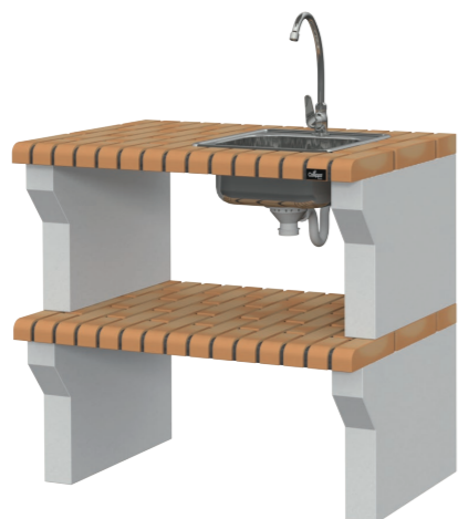
BATALHA MT92LL2 // 92L x 58P x 86A cm. // Kg 220 // LL2 - Dim: 38 x 38 cm.
