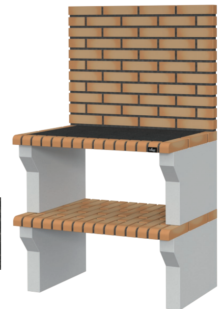
BATALHA MT92GPT // 92L x 58P x 155A cm. // Kg 285
