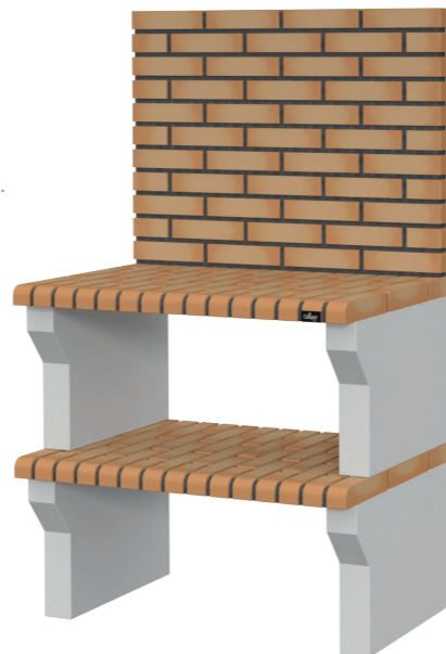
BATALHA MT92PT // 92L x 58P x 155A cm. // Kg 285
