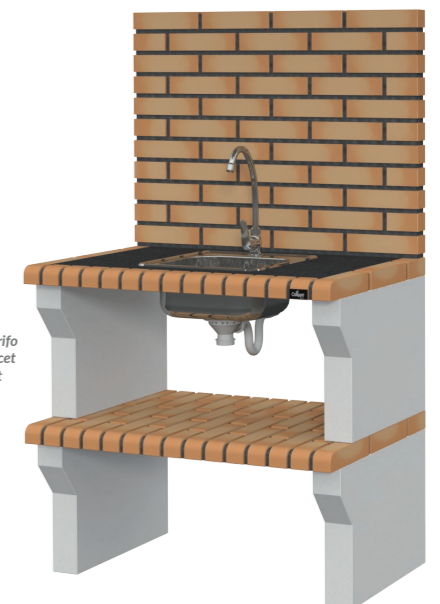
BATALHA MT92GLL2PT // 92L x 58P x 155A cm. // Kg 285 // LL2 - Dim: 38 x 38 cm.
